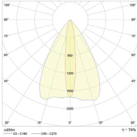
CREE J3030
