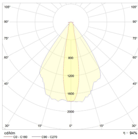
CREE J3030
